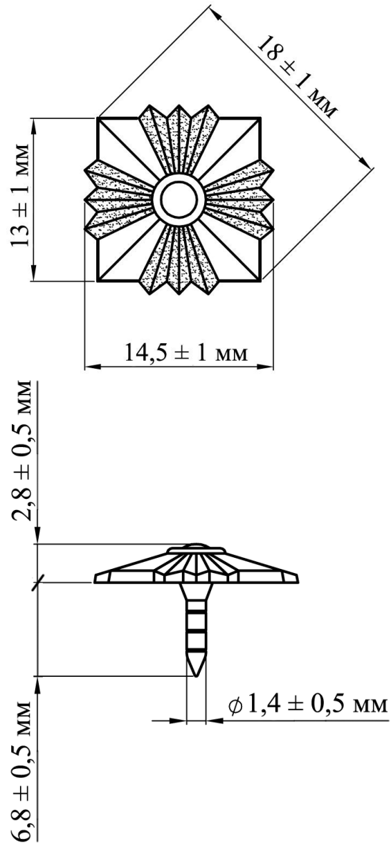
Рисунок Д1.1 – Розміри предмета
